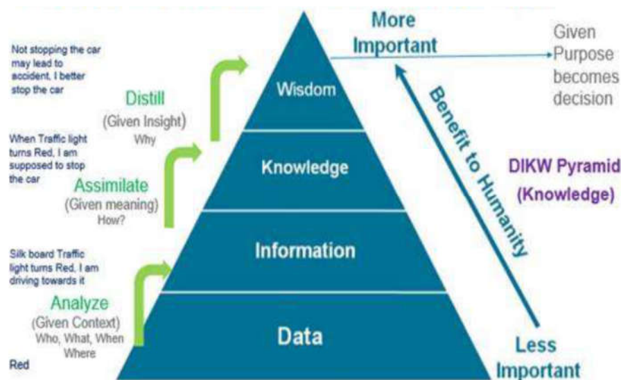
Fig. 4 DIKW pyramid
